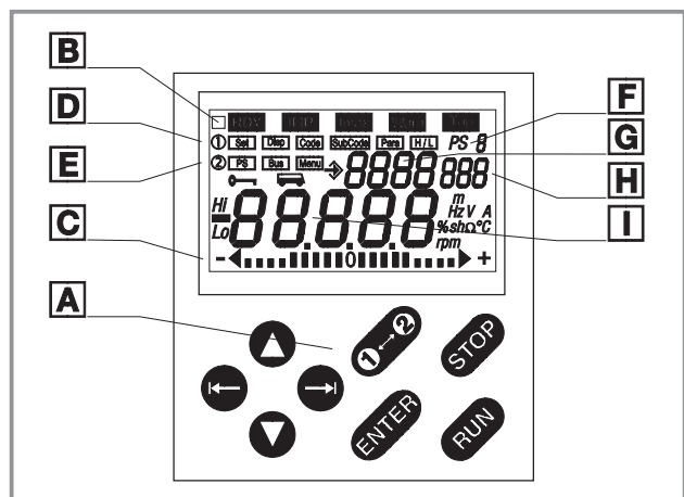
Keypad
